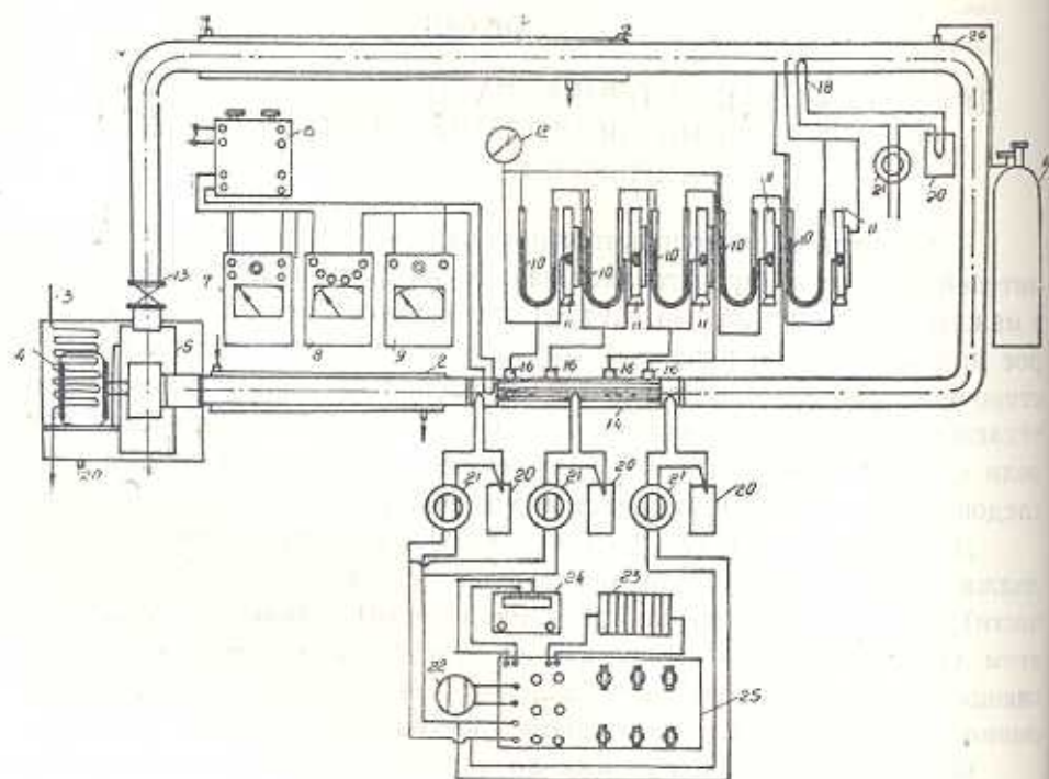
Рис. 1. Принципиальная схема экспериментальной установки: 1—аэродинамическая труба, 2—холодильник, 3—охлаждение двигателя, 4—электродвигатель, 5—вентиль, 6—трансформатор, 7—ваттметр, 8—амперметр, 9—вольтметр, 10—дифманометр, 11—микроманометр, 12—манометр, 13—задвижка, 14—экспериментальный участок, 15—пневмометрическая трубка, 16—отборник статического давления, 17—баллон, 18—пятиспайные термобатарей, 19—термопары на поверхности, 20—сосуд Дюара, 21—переключатель, 22—нормальный элемент, 23—аккумулятор, 24—гальванометр, 25—потенциометр, 26—штуцер.
