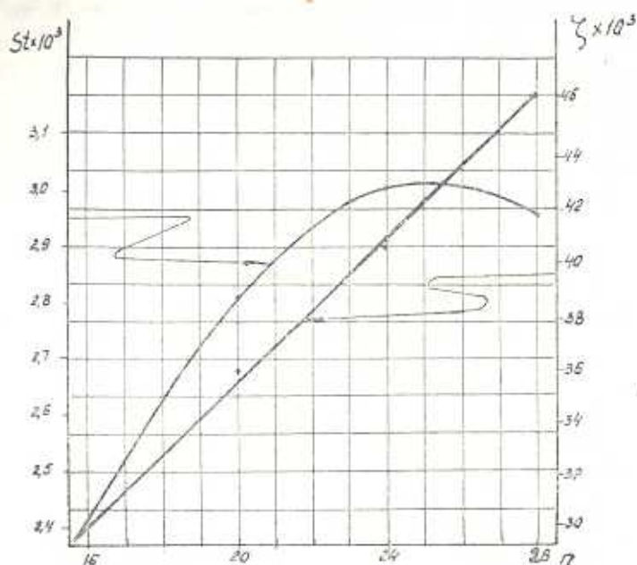
Рис. 4. Зависимость интенсивности теплообмена и гидродинамического сопротивления от числа ребер при R_c = 4 \cdot 10^4 ( h = 10 мм; d = 48 мм; D = 107 мм).
