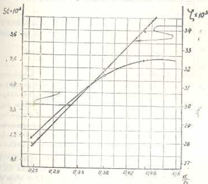
Рис. 3. Зависимость интенсивности теплообмена и гидродинамического сопротивления от диаметра несущей трубы при Re = 4 \cdot 10^4 ( n = 20 мм, h = 10 мм; D = 107 мм).
