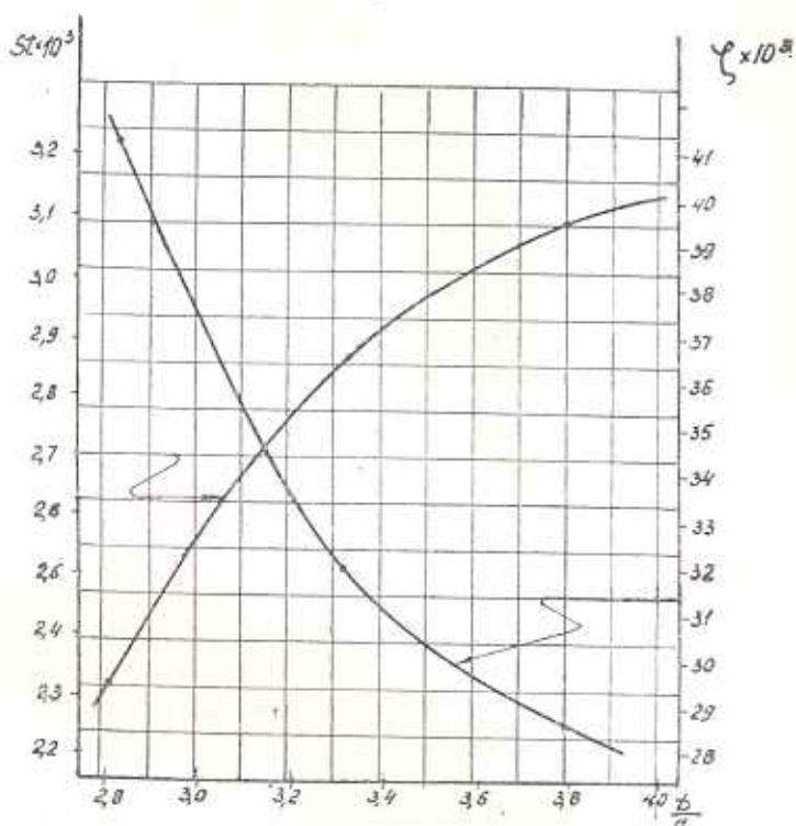
Рис. 2. Зависимость интенсивности теплообмена и гидродинамического сопротивления от диаметра канала при R_c^* = 4 \cdot 10^4 ( d = 28 мм; n = 20 ; h = 10 мм).
