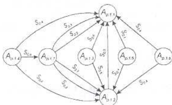
Рис. 4. Матрица и граф процесса сборки реле верхнего уровня
