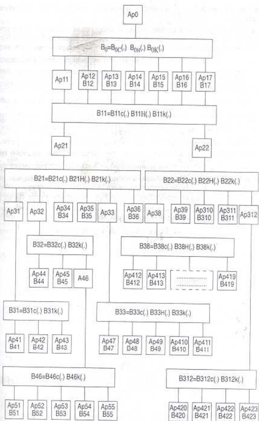
Рис. 3. Иерархическая структура построения электромагнитных реле поворотного типа
