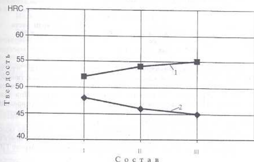
Рис. 2. Зависимость твердости поверхности (кривая 1) и сердцевины (кривая 2) стали 40X от состава
