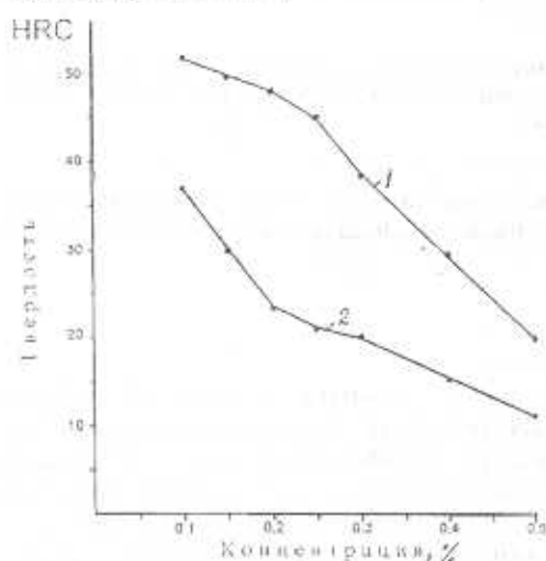
Рис. 1. Зависимость твердости поверхности (кривая 1) и сердцевины (кривая 2) стали 40X от концентрации
